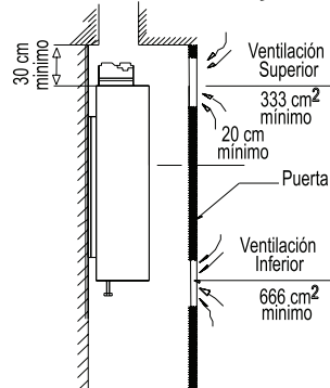
montaje en un closet
