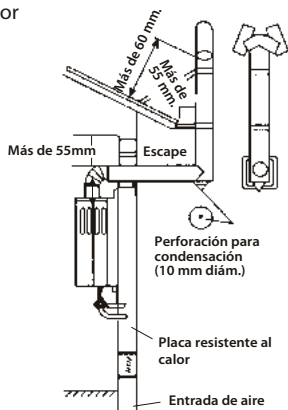
Esquema de dibujo para la instalación de tubería de combustión independiente
