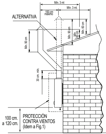
instalación en exteriores
